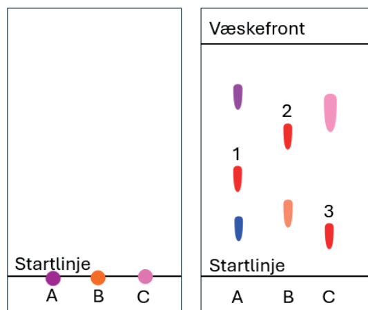
Figur 1. Tynnsjiktplate før og etter kromatograferingen
