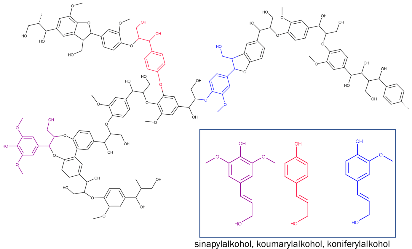
Figur 11. Utsnitt av strukturen til lignin (øverst og til venstre) og monomerane (i høgre hjørne)
